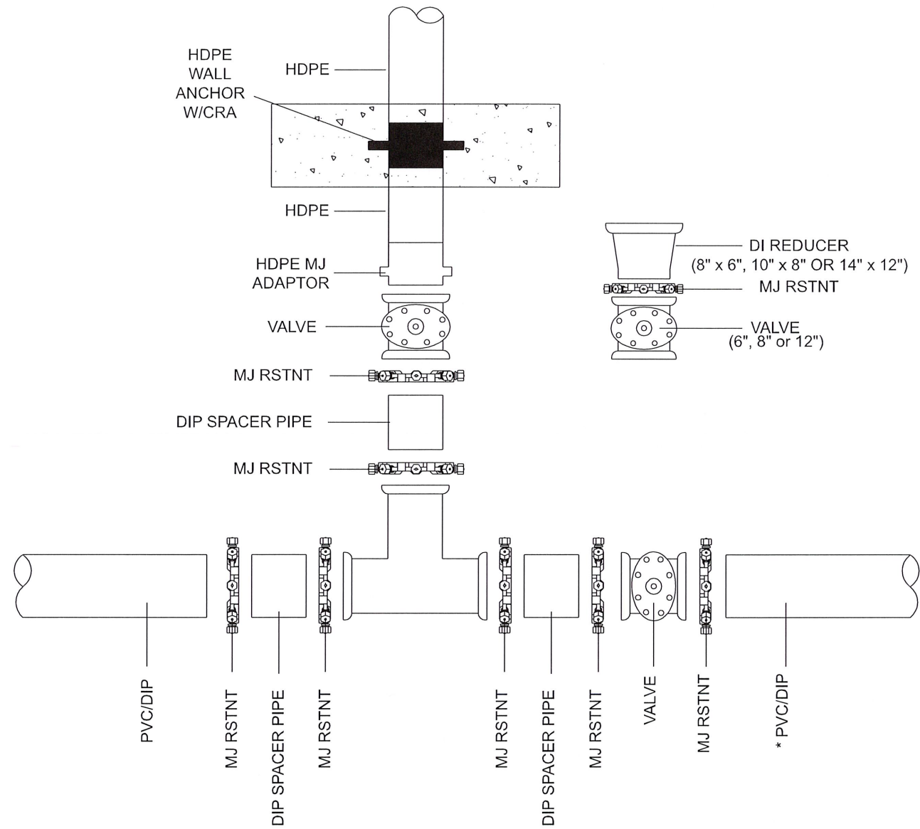
DI TEE (DI MAIN / HDPE BRANCH)
